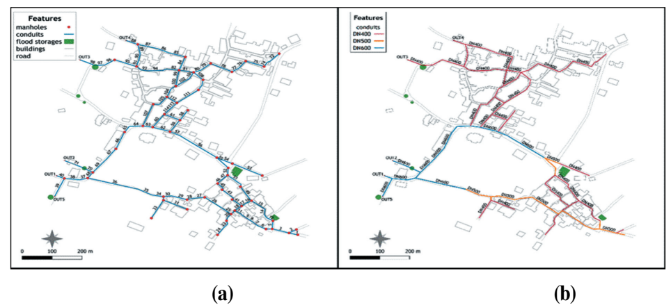
Εικόνα 3: Συνοπτικά διαγράμματα του προτεινόμενου δικτύου (α) οι σωλήνες με τα φρεάτια και οι έξοδοι του συστήματος και (β) η διαστασιολόγηση του δικτύου.
