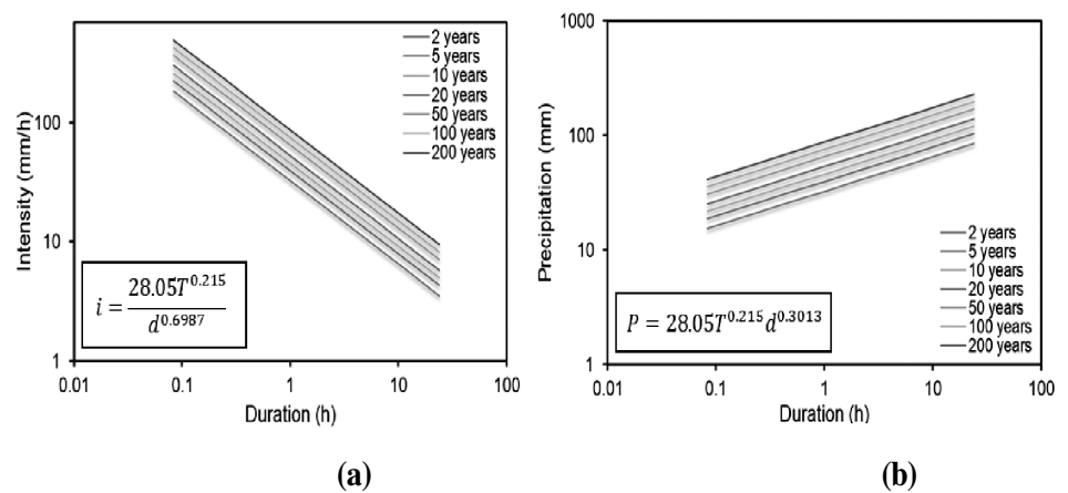
Εικόνα 2: (α) Όμβριες καμπύλες (b) και καμπύλες ύψους βροχοπτώσης για την Φουρνή, με περίοδο επαναφοράς 2, 5, 10, 20, 50, 100 και 200 χρόνια.
