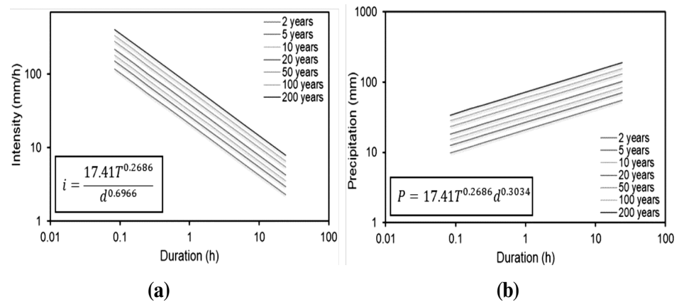
Εικόνα 1: (α) Όμβριες καμπύλες (b) και καμπύλες ύψους βροχοπτώσης για το Ηράκλειο, με περίοδο επαναφοράς 2, 5, 10, 20, 50, 100 και 200 χρόνια.
